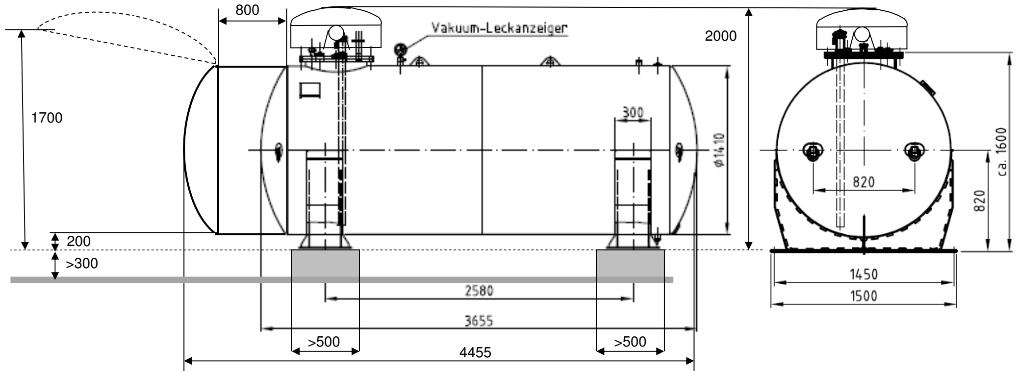
Flugfeldtankanlage CT 5000 de luxe Ausrüstung in eichfähiger oder nicht eichfähiger Ausführung, alle Armaturen und Schlauchleitungen im de luxe- Schrank
